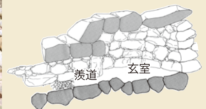
横穴式石室模型図
